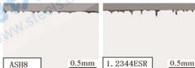
3000次下热疲劳试样截面形貌
