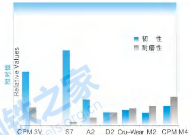
工具钢韧性和耐磨性对照表
