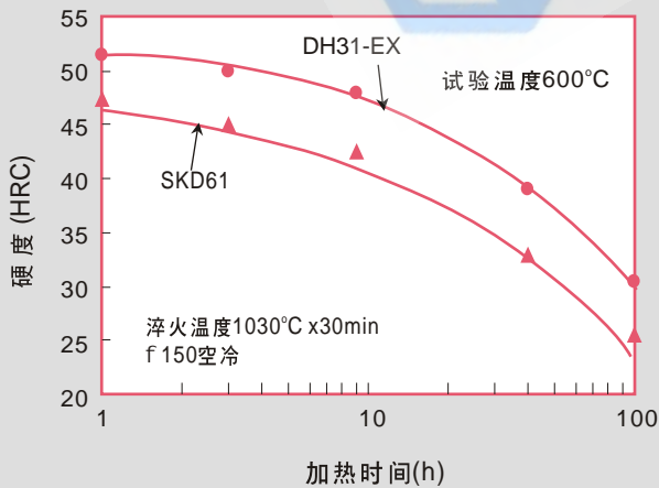
DH31-EX的高温特性
